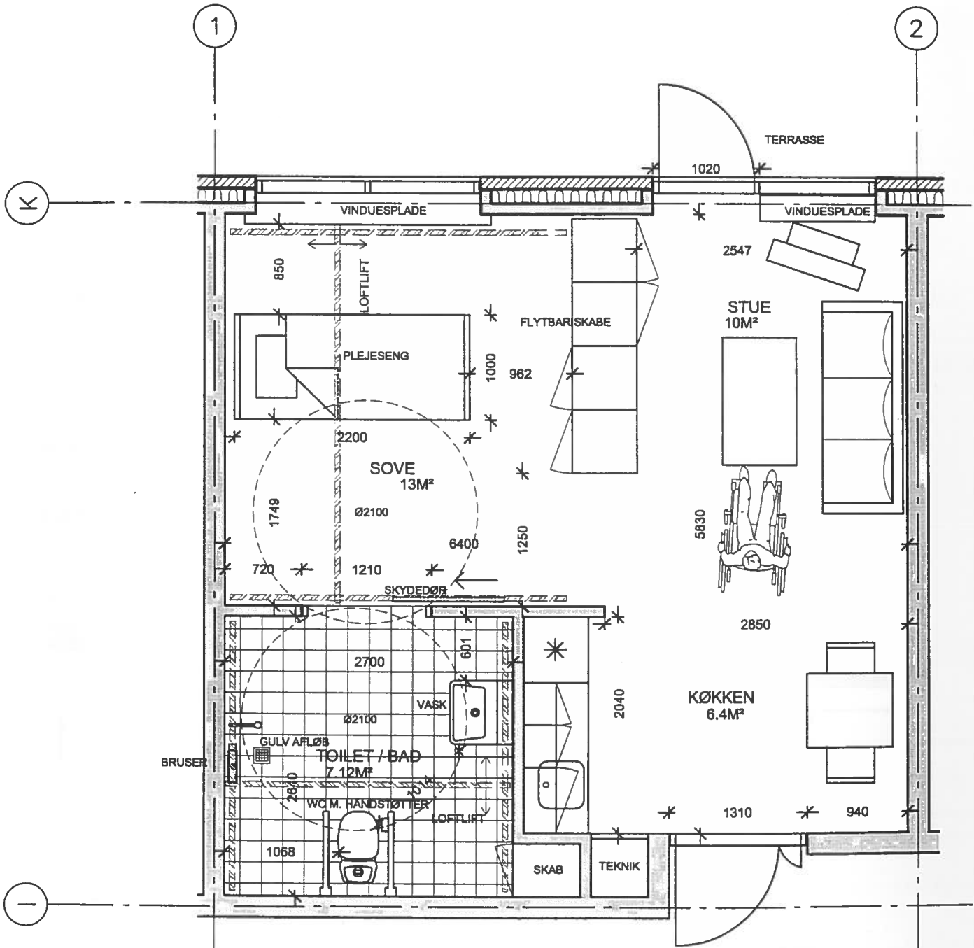
BOLIGPLAN
