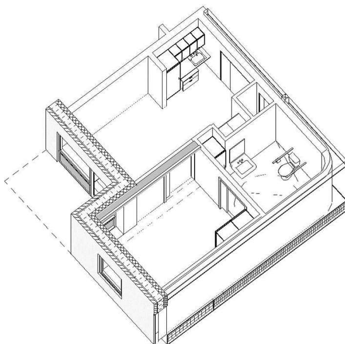
2-rums lejlighed (type A, B ,C + D)
