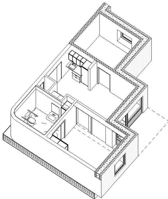
3-rums lejlighed (type E)
